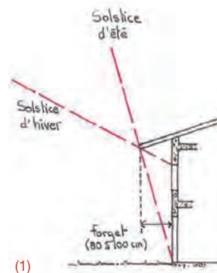
Le forget débordant, une protection simple contre le soleil d'été (1) et la pluie (2)
