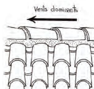
Position des tuiles de faîtage
