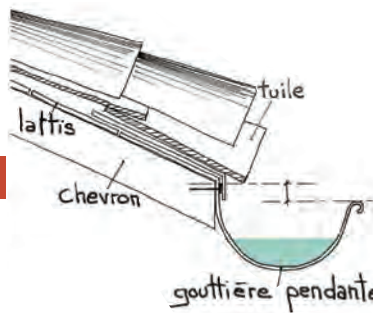
Mise en oeuvre d'une gouttière pendante
