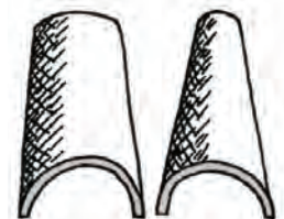
Tuile «droite» et tuile «gironnée»
